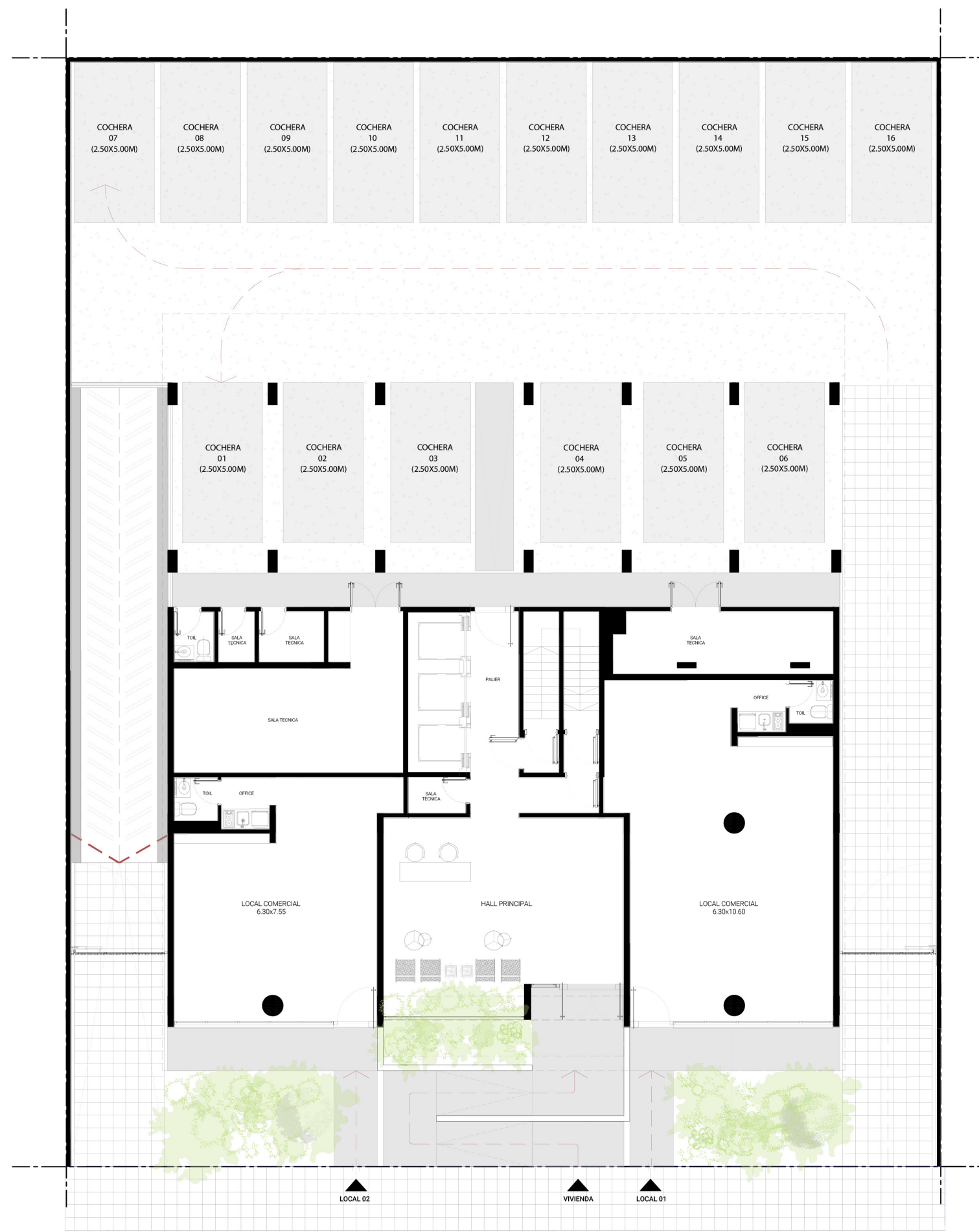
Planta Baja
